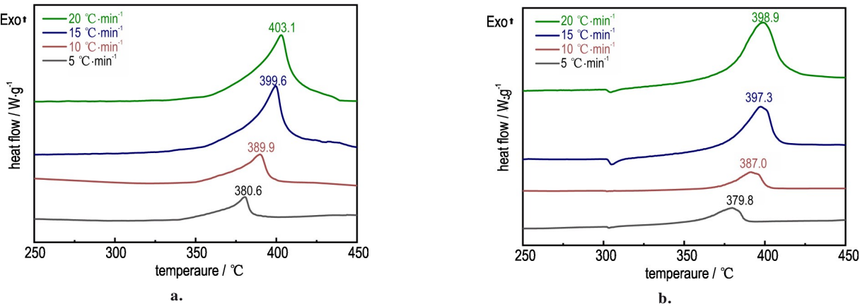
图 3 DPE-1 和 PAP-2 的 DSC 曲线 Fig.3 DSC curves of DPE-1 and PAP-2
