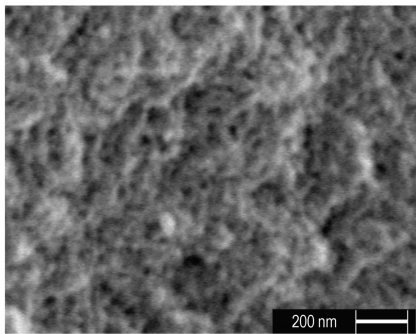
图3 RDX/RF 纳米复合含能材料的 SEM 图
