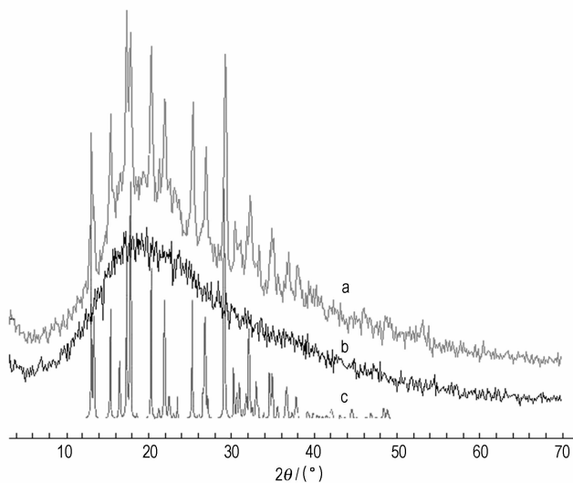
图5 RDX/RF(a), RF(b), RDX(c) 的衍射图
