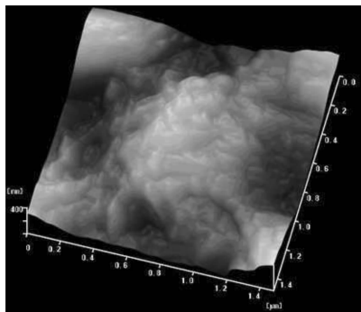
图4 RDX/RF 纳米复合含能材料的 AFM 图
