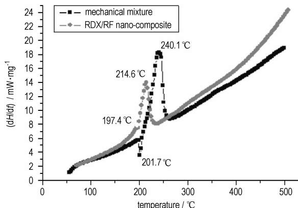
图6 RF 与 RDX 机械混合物和 RDX/RF 复合物的 DSC 曲线
